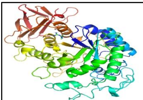
4W93 metformin
